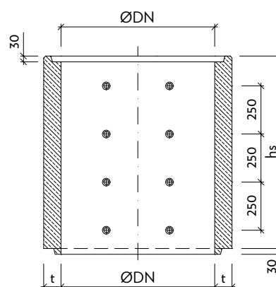
LS14 - STUDNIČNÍ A DRENÁŽNÍ SKRUŽE DN 1000, t 90
