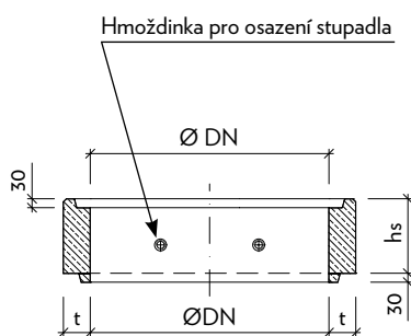
LS11 - STUDNIČNÍ A DRENÁŽNÍ SKRUŽE DN 800, t 90
