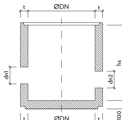
LS15 - STUDNIČNÍ A DRENÁŽNÍ DNA DN 1000, t 90 LS12 - STUDNIČNÍ A DRENÁŽNÍ DNA DN 800, t 90
