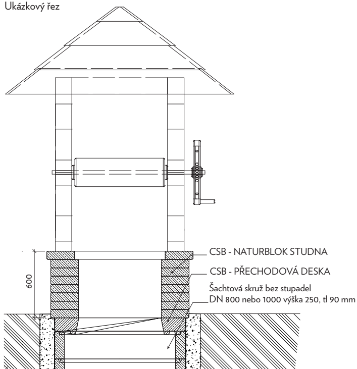
Ukázkový řez
