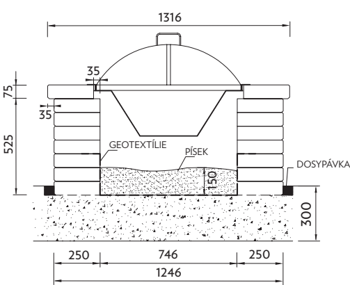
ukázkový řez
