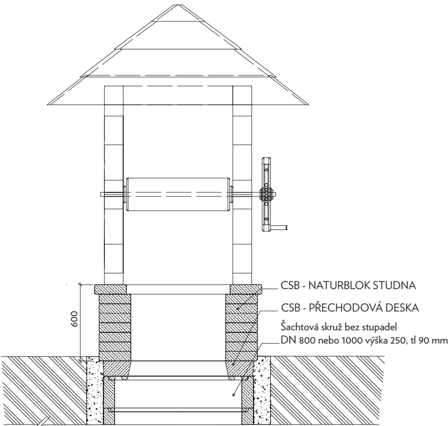
ukázkový řez
