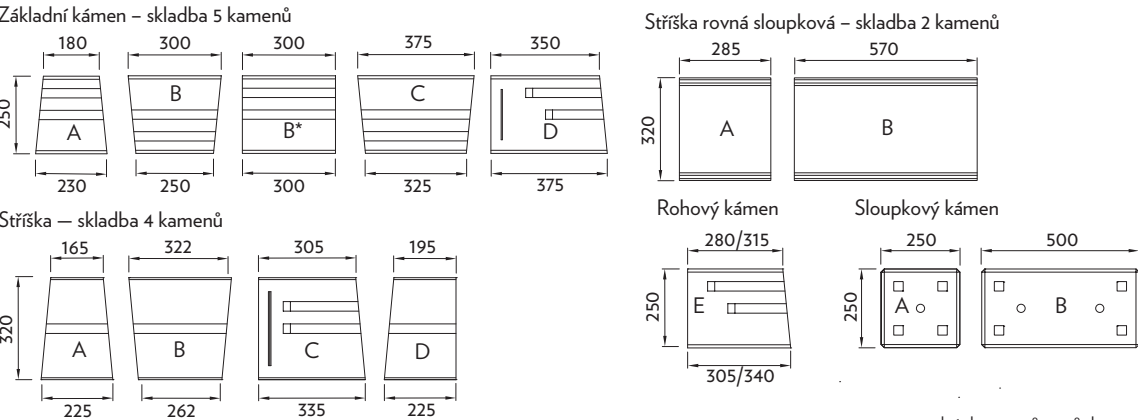
ukázka tvarů - půdorys
