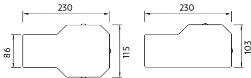
ukázka tvaru - půdorys
