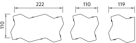
ukázka tvaru - půdorys
