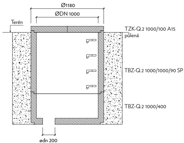
Studna vrtaná
