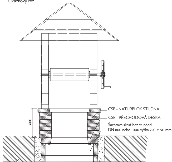
Ukázkový řez
