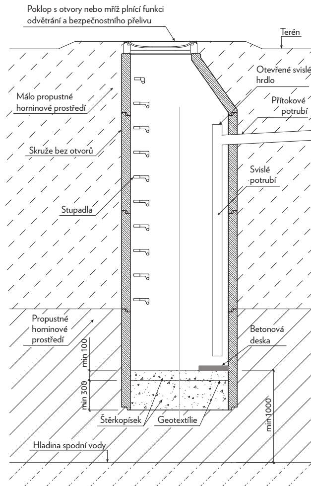
Vsák
