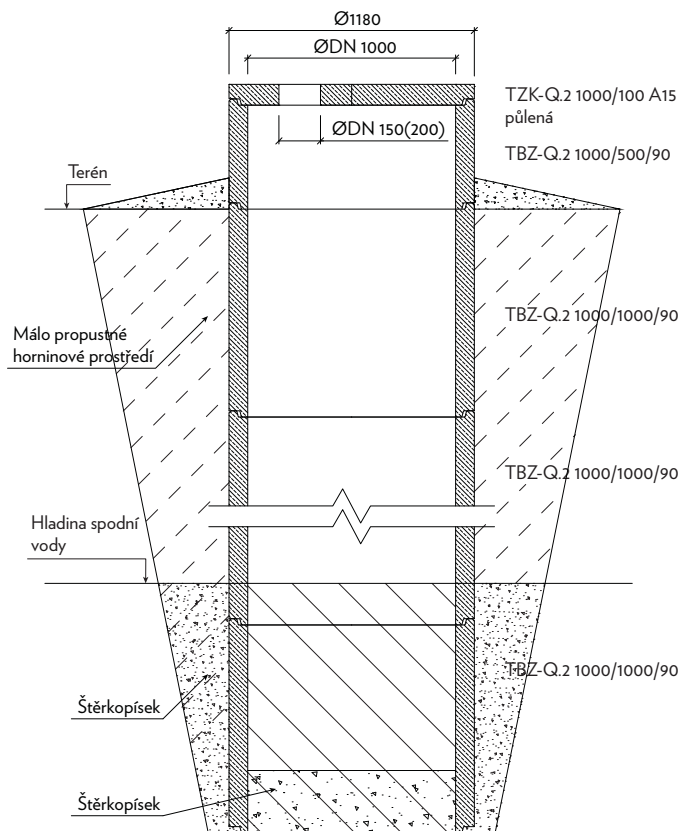
Studna kopaná
