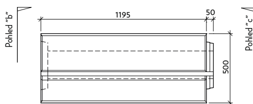
Půdorys
