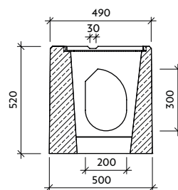
Řez: b-b'
