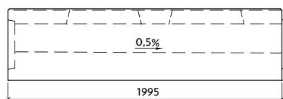
Profil VII-1-G20/21-L s vnitřním spádem
