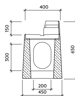
Řez: b-b' I-4-V0
