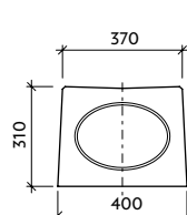
Pohled "b" T-ZU - pero
