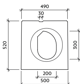
Pohled "a" VII-0-VU - drážka
