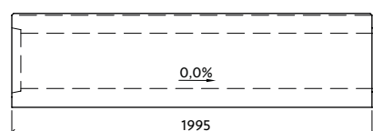
Profil VII-4-T30/30-L bez vnitřního spádu
