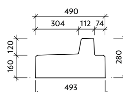
Pohled "b" VII-3-O
