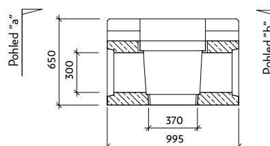
Řez: a-a' I-6-VU
