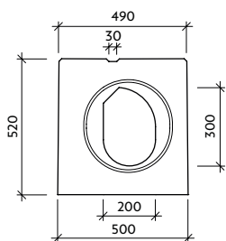
Pohled "b" VII-1-V0-L - pero
