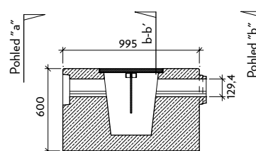
Řez: a-a' T-0-PP
