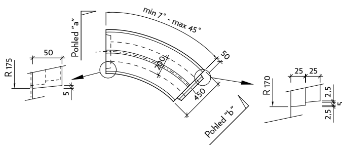
Půdorys
