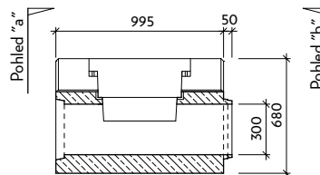
Řez: a-a' I-7-C0
