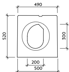
Pohled "a" VII-1-C0-L - drážka
