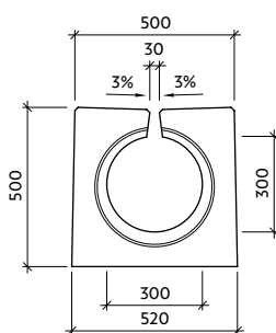
Pohled "b" II-1-V0 - pero
