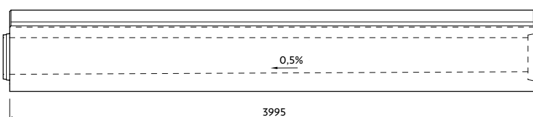
Profil I-3-G26/28-L se spádem dna
