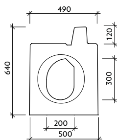
Pohled "a" VII-3-C0-L - drážka
