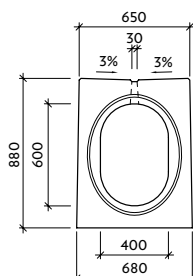
Pohled "a"="b" VI-1-CS - pero/pero
