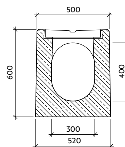
Řez: b-b' III-0-C0
