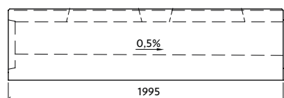
Profil VII-1-G22/23-L s vnitřním spádem
