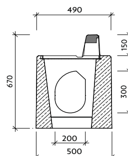
Řez: b-b'
