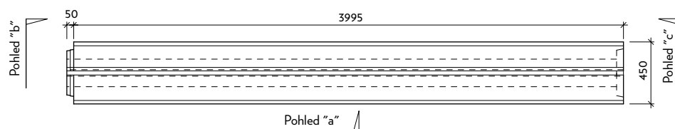
Půdorys
