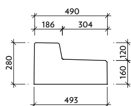
Pohled "b" VII-3-O-12-0
