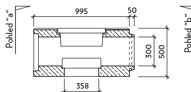
Řez: a-a' II-0-V0
