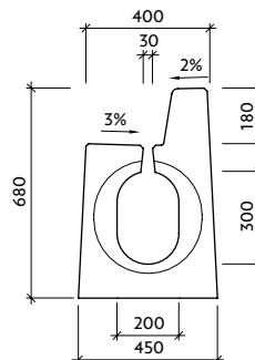
Pohled "b" I-0-7 - drážka
