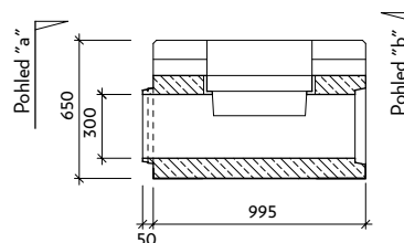
Řez: a-a' I-4-C0
