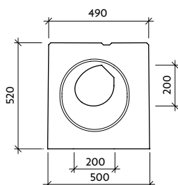
Pohled "b" VII-0-CS - pero
