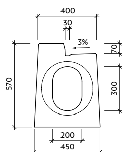
Pohled "a" I-2-VU - drážka/drážka
