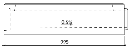
Profil M-G 135/140 se spádem dna
