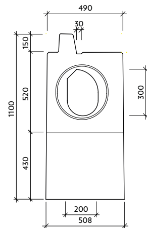
Pohled "b" VII-3-PP-L - pero
