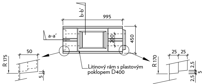
Půdorys
