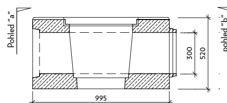
Řez: a-a' VII-0-L
