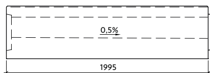
Profil VII-0-G20/21-P s vnitřním spádem
