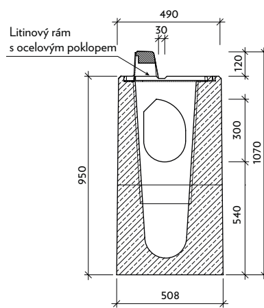
Řez: b-b' VII-3-PP-L
