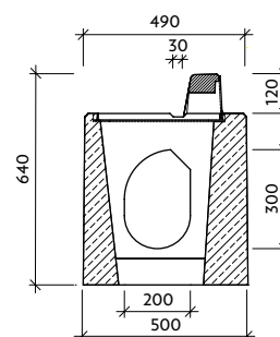
Řez: b-b'
