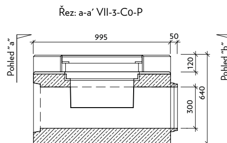
Profil VII-3-C0-P - čistící kus základní pravý
