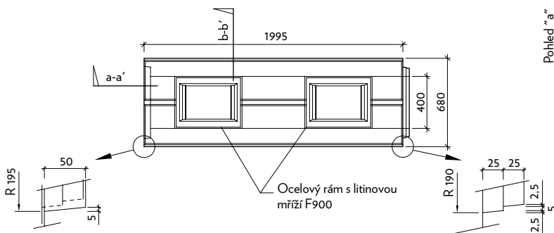
Půdorys
