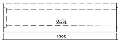
Profil VII-0-G29/30-L s vnitřním spádem
