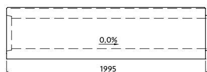
Profil VII-4-T30/30-P bez vnitřního spádu
