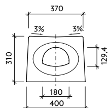
Pohled "a" T-1-C0 - drážka
