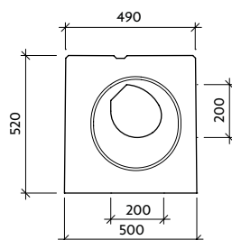
Pohled "a" VII-0-CS - pero
