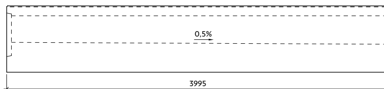
Profil IV-0-G28/30 se spádem dna
