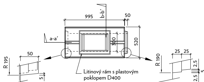
Půdorys
