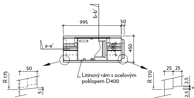
Pūdorys
