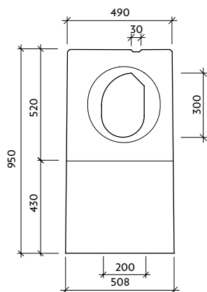
Pohled "a" VII-1-PP-L - drážka
