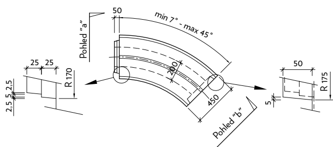
Půdorys
