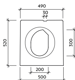
Pohled "a" VII-1-V0-L - drážka
