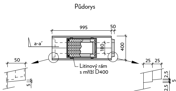
T-1-V0 - vpusťový kus základní s litinovou mříží pro zatížení D400
