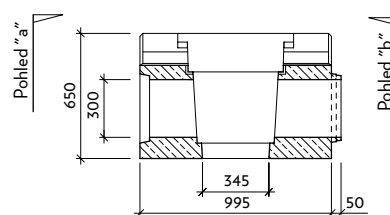
Řez: b-b' I-4-V0
