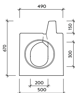
Pohled "b" VII-4-P-C0 - pero
