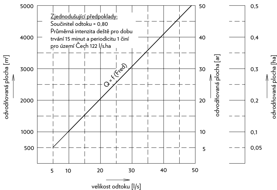
NOMOGRAM č. 2
