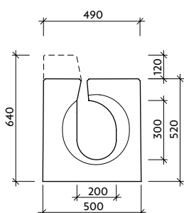
Pohled "b" - drážka
