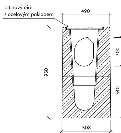
Řez: b-b' VII-1-PP-P
