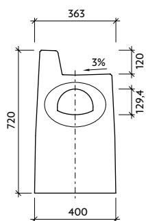
Pohled "a" T-3-PP - drážka
