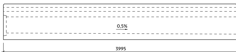
Profil I-5-G28/30-P se spádem dna
