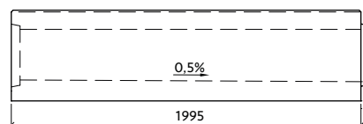
Profil VII-3-G29/30-P s vnitřním spádem
