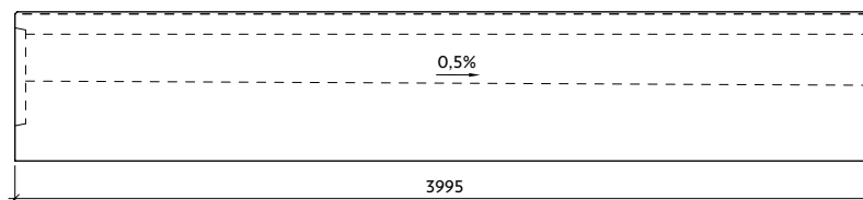
Profil IV-0-G22/24 se spádem dna
