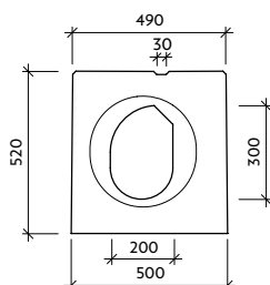
Pohled "a" VII-0-V0-L - drážka
