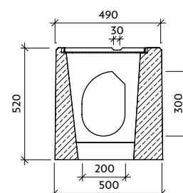
Řez: b-b'
