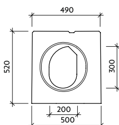
Pohled "b" VII-0-C0-P - pero
