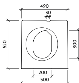
Pohled "b" VII-I-VU - drážka
