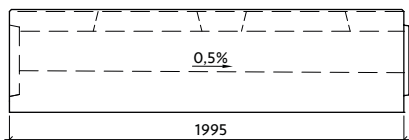
Profil VII-1-G20/21-P s vnitřním spádem
