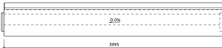
Profil I-3-T20/20-L bez vnitřního spádu
