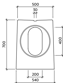
Pohled "b" IV-1-C0 - pero
