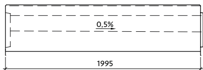
Profil VII-3-G20/21-P s vnitřním spádem
