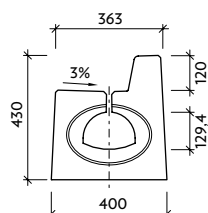
Pohled "b" T-0-3-P - pero
