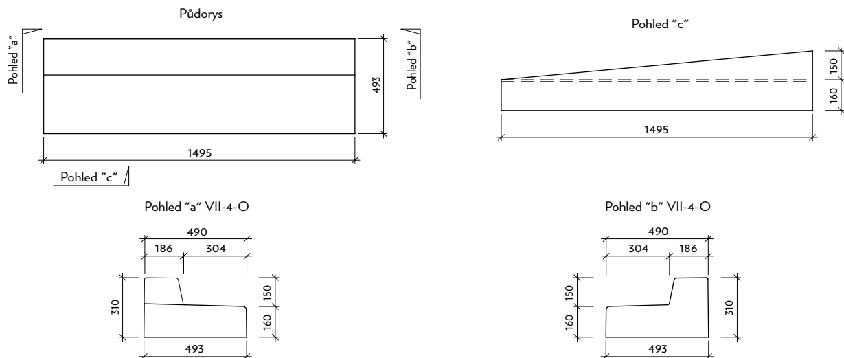
Profil VII-4-O tunelový obrubník (náběh 0-15cm)
