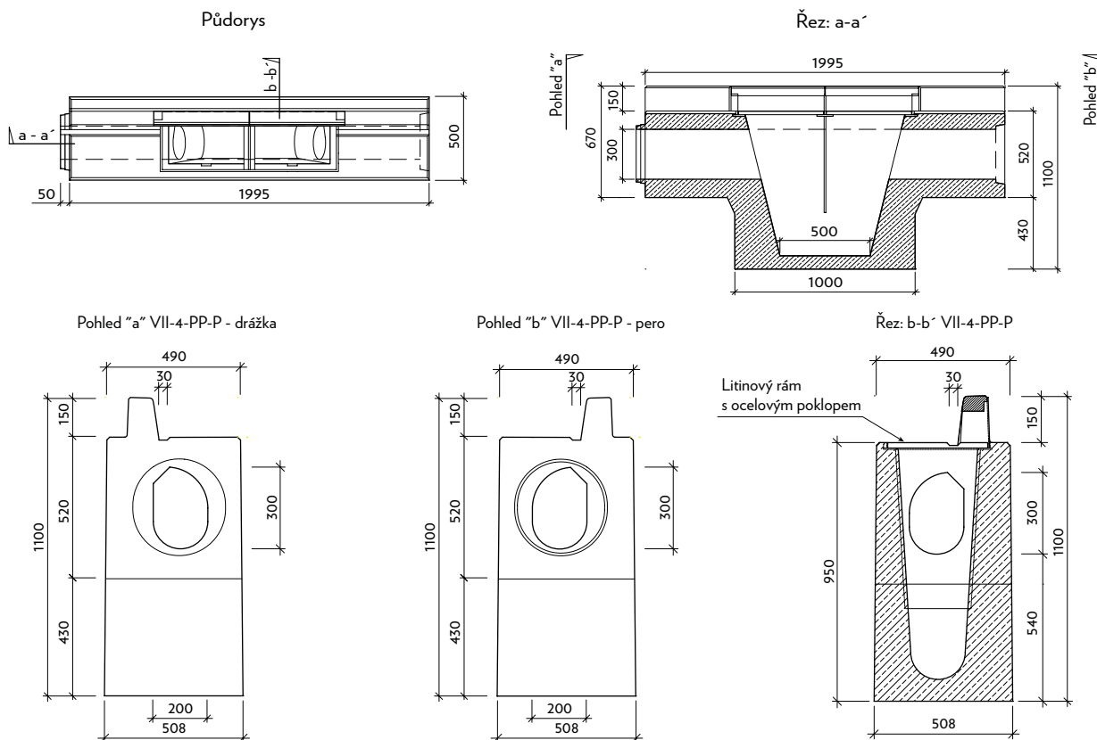
Profil VII-4-PP - pravý - bezpečnostní protipožární uzávěra
