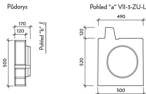
VII-3-ZU-L - záslepka pero levá
