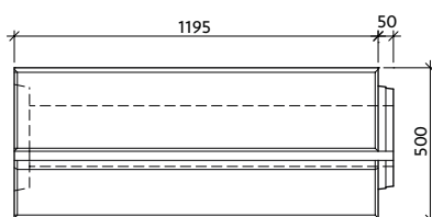
Podélný řez
