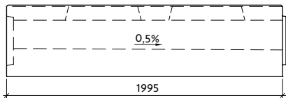
Profil VII-1-G21/22-P s vnitřním spádem
