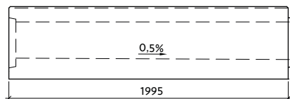
Profil VII-0-G21/22-L s vnitřním spádem
