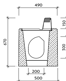
Řez: b-b'
