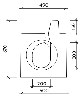
Pohled "b" V-4-L-V0 - drážka
