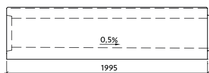
Profil VII-4-G29/30-P s vnitřním spádem
