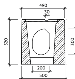
Řez: b-b'
