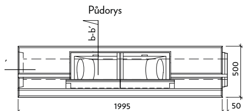
Profil VII-4-PP - levý- bezpečnostní protipožární uzávěra
