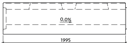
Profil VII-1-G25/26-P bez vnitřního spádu
