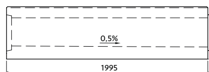
Profil VII-3-G28/29-P s vnitřním spádem
