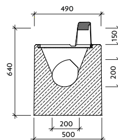
Řez: b-b'
