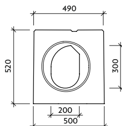
Pohled "b" VII-I-C0-P - pero
