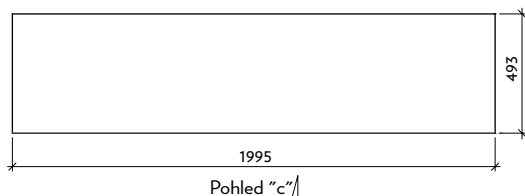
Půdorys
