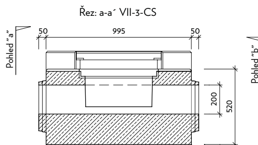
VII-3-CS čistící kus vrcholový
