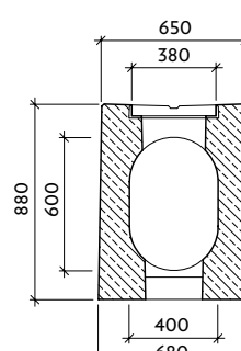
Řez: b-b'
