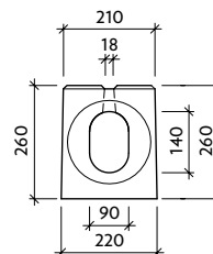
Pohled "b" M roh 90° - drážka
