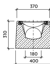
Řez: b-b' T-1-CS
