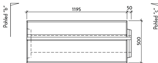
Podélný řez
