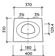
Pohled "a" T-1-VU - drážka/drážka
