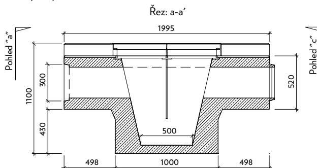
Profil VII-4-PP - levý- bezpečnostní protipožární uzávěra
