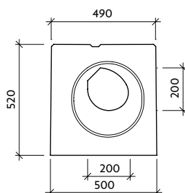
Pohled "a" VII-I-CS - pero
