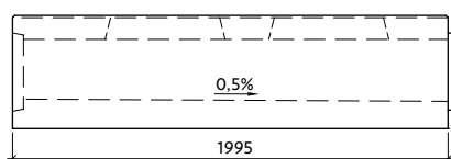
Profil VII-1-G28/29-P s vnitřním spádem
