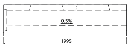
Profil VII-1-G24/25-L s vnitřním spádem
