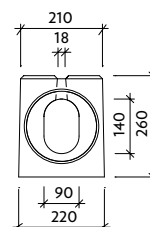
Pohled "b" M roh 90° - pero
