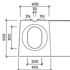
Pohled "a" - drážka
