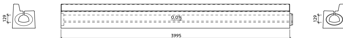
Profil T-3-T13/13 bez vnitřního spádu
