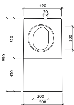
Pohled "b" VII-1-PP-P - pero
