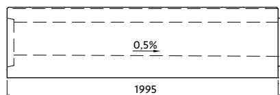
Profil VII-4-G24/25-L s vnitřním spádem
