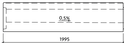
Profil VII-4-G21/22-P s vnitřním spádem
