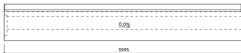
Profil I-3-T22/22-P bez vnitřního spádu
