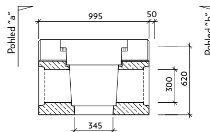
Řez: a-a' I-7-VU
