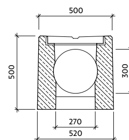
Řez: b-b' II-1-V0
