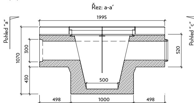
Profil VII-3-L - protipožární přepážka levá
