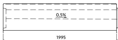
Profil VII-3-G20/21-P s vnitřním spádem
