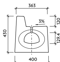
Pohled "a" T-3-0-P - drážka
