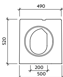
Pohled "b" VII-0-C0-P - pero
