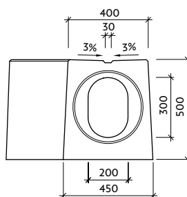
Pohled "a" - pero
