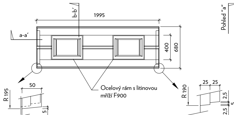
Pohled "a"="b" VI-1-VU - drážka/drážka
