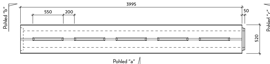
Půdorys
