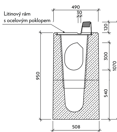
Řez: b-b' VII-3-PP-P
