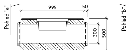
Řez: a-a'
