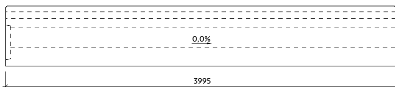
Profil I-5-T20/20-P bez vnitřního spádu
