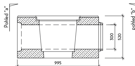
Řez: a-a' VII-0-P
