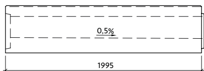
Profil VII-3-G21/22-P s vnitřním spádem
