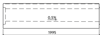
Profil VII-4-G26/27-P s vnitřním spádem
