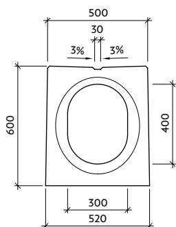
Pohled "a" III-1-V0 - drážka
