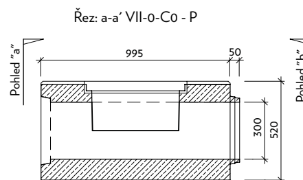
VII-0-C0-P - pravý čistící kus základní
