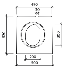
Pohled "b" VII-1-V0-P - pero
