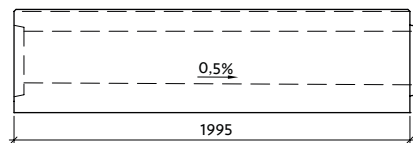
Profil VII-3-G26/27-L s vnitřním spádem
