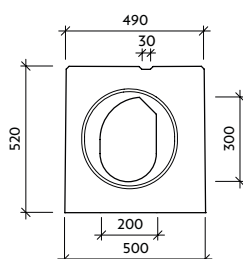
Pohled "b" VII-0-V0-P - pero
