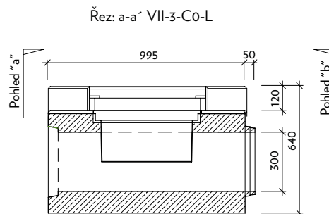
Profil VII-3-L - čistící kus základní levý
