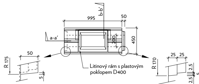
Půdorys
