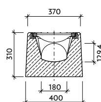
Řez: b-b' T-0-CS
