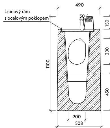
Řez: b-b' VII-3-PP-L
