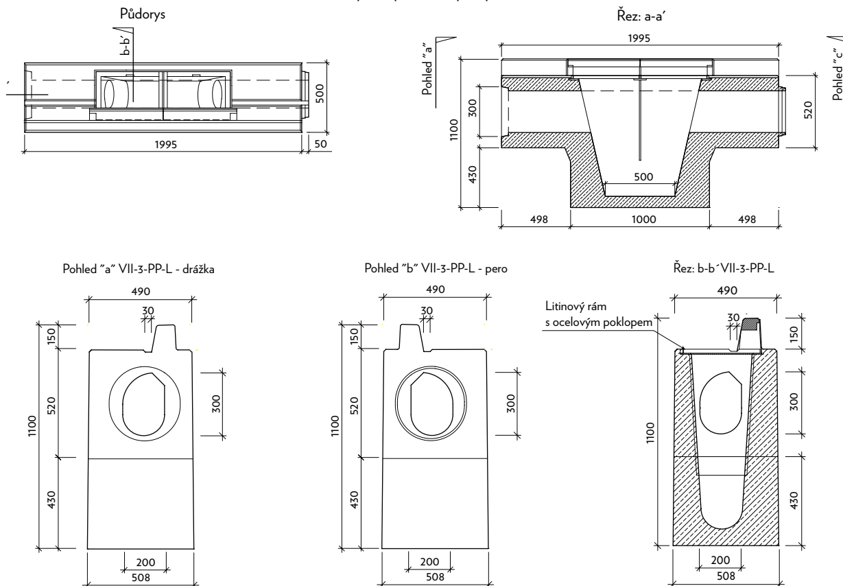
Profil VII-4-PP - levý - bezpečnostní protipožární uzávěra
