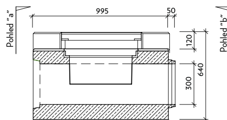
Řez: a-a' VII-3-C0-L
