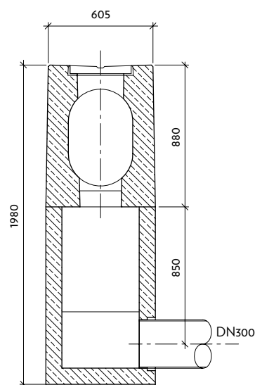
Řez: b-b'
