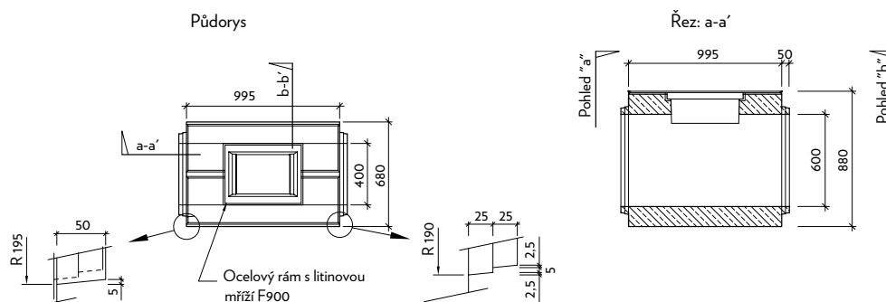
VI-1-CS - čistící kus vrcholový s ocelovým rámem a litinovou mříží pro zatížení F900
