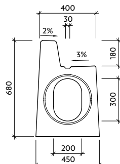
Pohled "a" I-7-0 - pero
