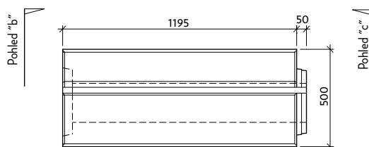
Půdorys
