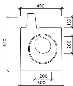
Pohled "a" VII-4-CS - pero
