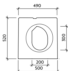
Pohled "a" VII-0-C0-P - drážka
