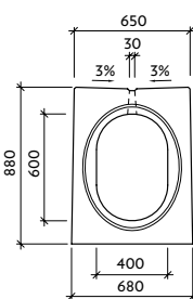
Pohled "b" VI-1-C0 - pero
