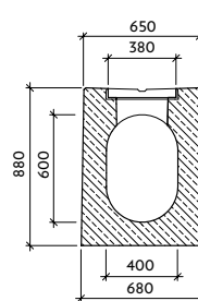
Řez: b-b'
