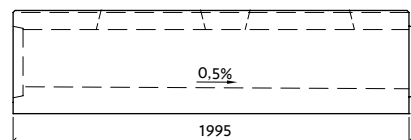
Profil VII-1-G28/29-L s vnitřním spádem
