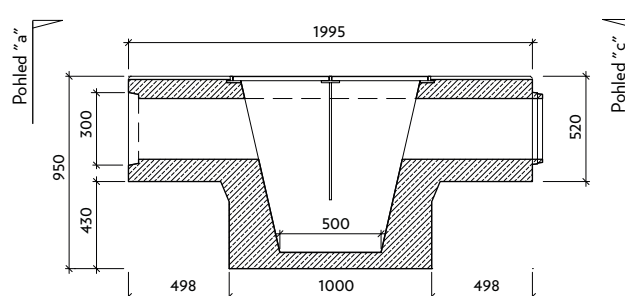
Pohled "b" VII-1-PP-L - pero
