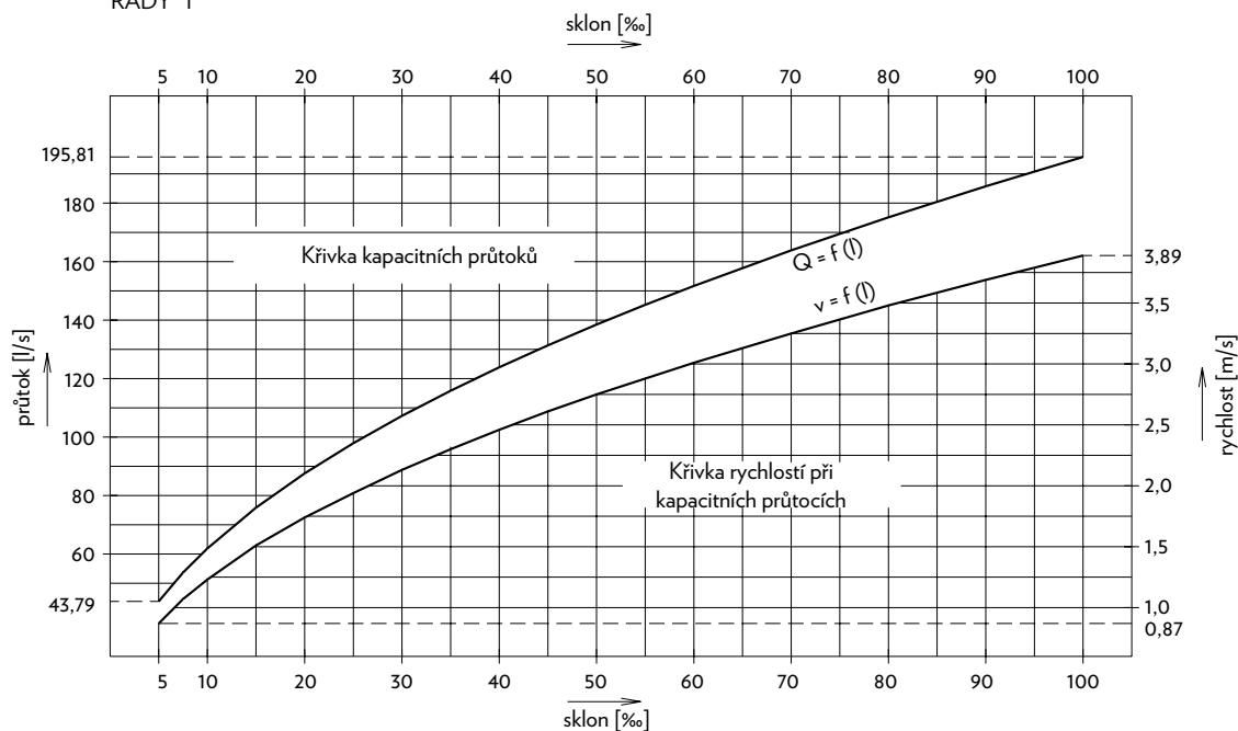
NOMOGRAM č. 1
