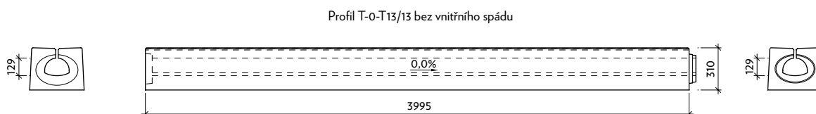
Pohled "b" T-0 - drážka
