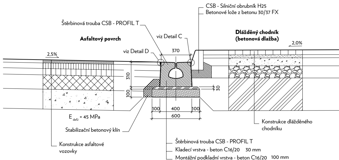
VZOROVÝ PŘÍČNÝ ŘEZ šterbinovým žlabem v komunikaci (PROFIL T, asfaltový povrch - obrubník, chodník)
