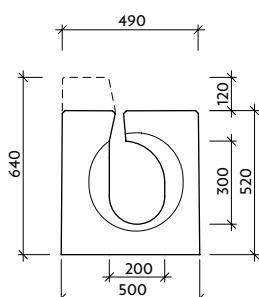
Pohled "b" - drážka
