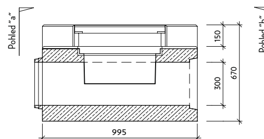
Řez: a-a' VII-4-C0-L
