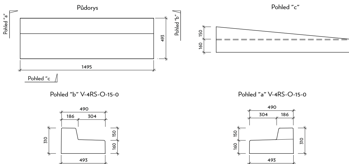
Profil VII-4-O - tunelový obrubník (náběh 15-0cm)
