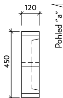
I-5-ZU - záslepka pero s obrubníkem 12 cm
