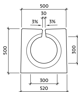
Pohled "a" II-1-C0 - drážka
