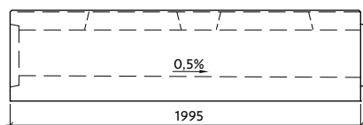
Profil VII-1-G27/28-P s vnitřním spádem
