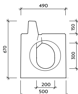
Pohled "a" VII-4-P-V0 - drážka
