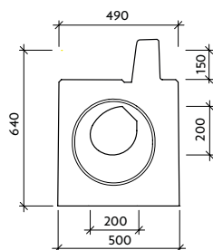
Pohled "b" VII-4-CS - pero
