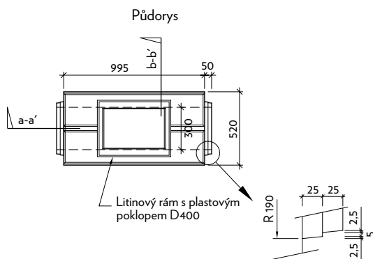
II-0-CS - čistící kus vrcholový s litinovým rámem a plastovým poklopem pro zatížení D400
