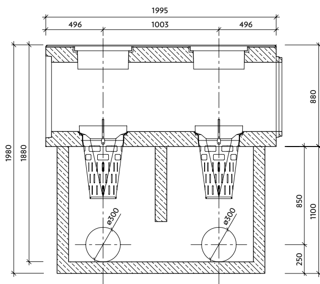
Řez: a-a'
