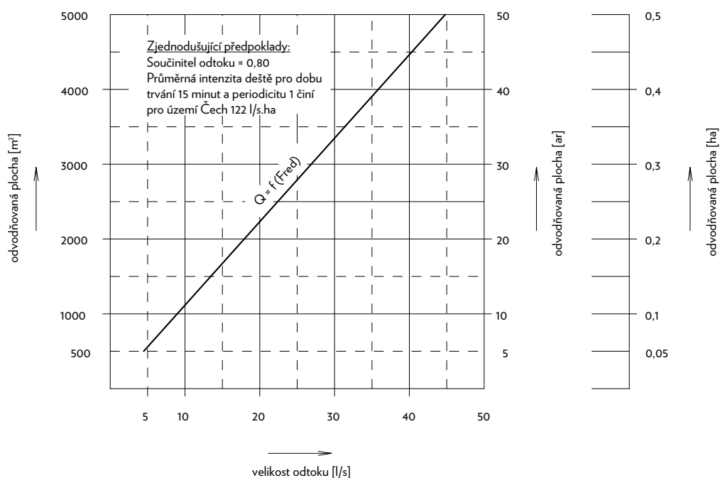
NOMOGRAM č. 2
