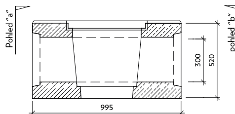
Řez: a-a' VII-0-VU
