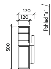
Půdorys VII-4-ZU - pravý
