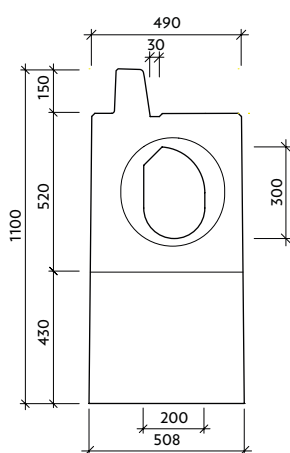
Pohled "a" VII-4-PP-P - drážka
