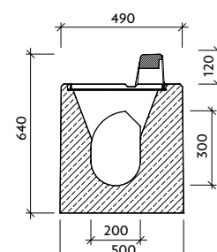
Řez: b-b'
