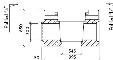
Řez: a-a' I-4-V0
