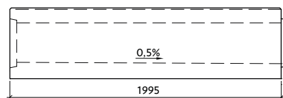
Profil VII-3-G29/30-L s vnitřním spádem
