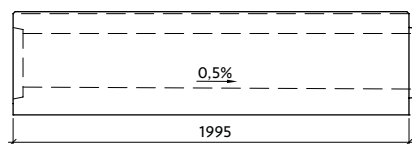
Profil VII-4-G27/28-P s vnitřním spádem
