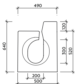
Pohled "b" - drážka
