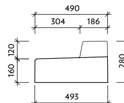
Pohled "a" VII-3-O-12-0
