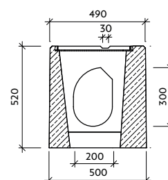
Řez: b-b'
