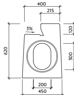
Pohled "b" I-5-V0 - pero
