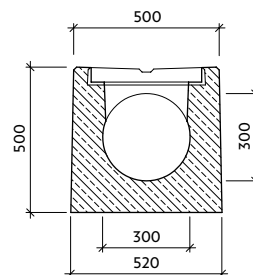
Řez: b-b' II-1-C0
