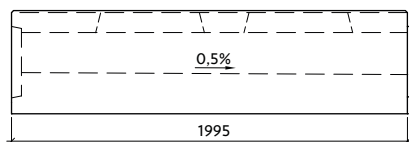
Profil VII-1-G21/22-L s vnitřním spádem
