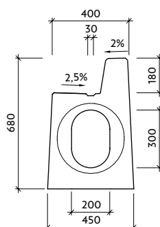
Pohled "b" I-7-V0 - drážka
