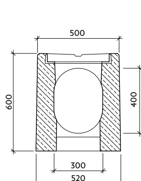
Řez: b-b'
