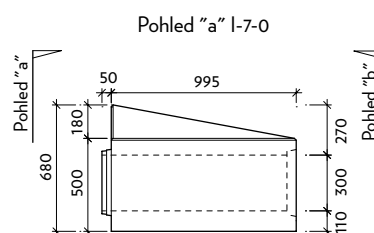
I-7-0 - levý - štěrbinová trouba s obrubníkem 18-0 cm náběhová
