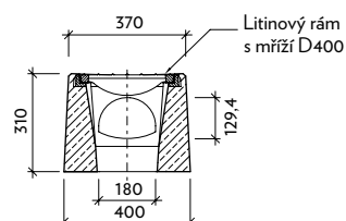
Řez: b-b' T-1-V0
