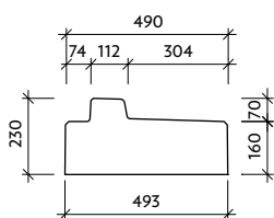
Pohled "a" VII-2-O
