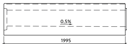
Profil VII-0-G26/27-L s vnitřním spádem
