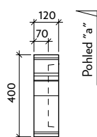
Půdorys T-3-ZZ levý
