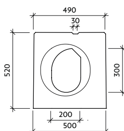
Pohled "b" VII-0-VU - drážka
