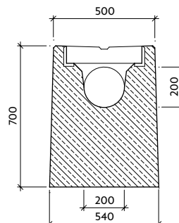
Řez: b-b' IV-1-CS
