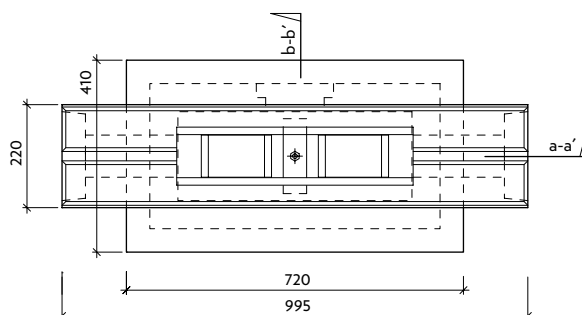
Půdorys
