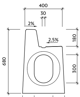
Pohled "a" I-7-VU - drážka/drážka
