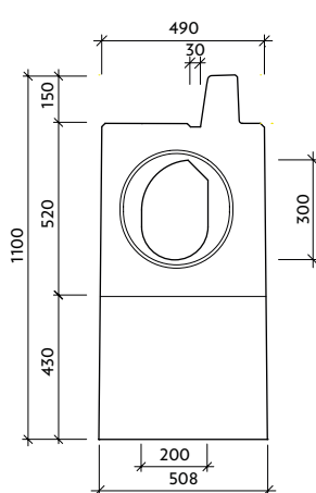
Pohled "b" VII-4-PP-P - pero
