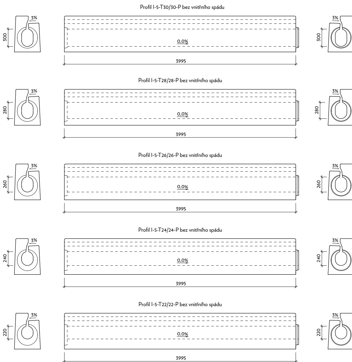
Pohled "b" I-5 - drážka
