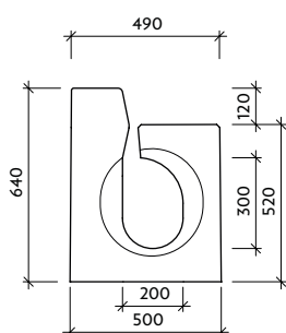
Pohled "b" - drážka
