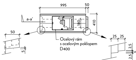
Půdorys
