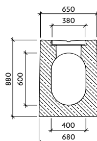
Řez: b-b'
