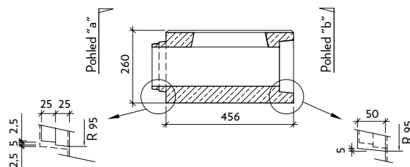
Řez: a-a' M roh 90° - levý
