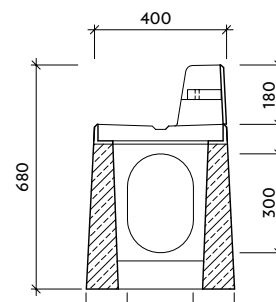
Řez: b-b' I-7-VU
