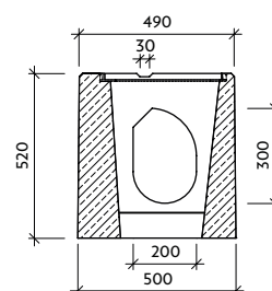
Řez: b-b'
