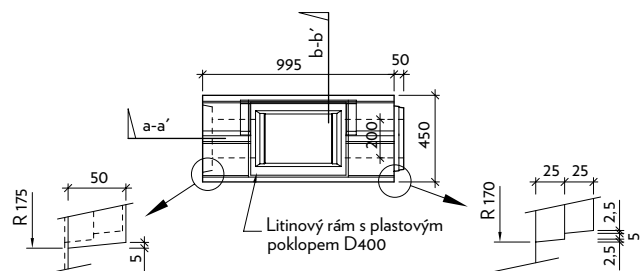
Půdorys
