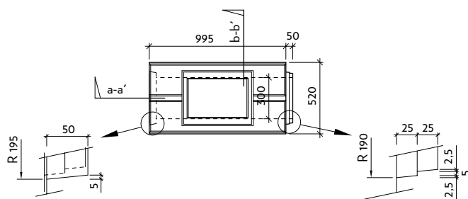
Půdorys
