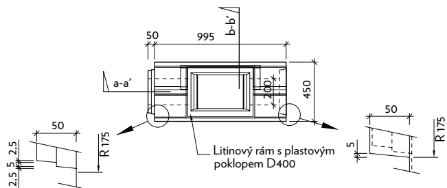
Půdorys
