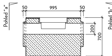
Řez: a-a' IV-1-CS
