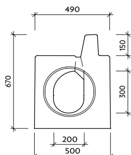
Pohled "b" VII-4-P-V0 - pero
