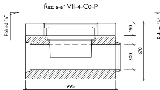
Profil VII-4-C0 - pravý - čistící kus, základní
