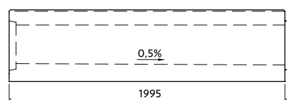
Profil VII-4-G28/29-P s vnitřním spádem
