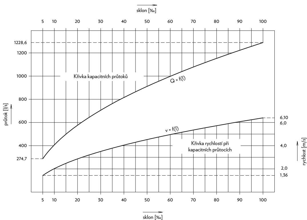
NOMOGRAM č. 2
