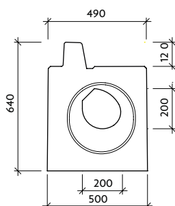
Pohled "a" VII-3-CS - pero
