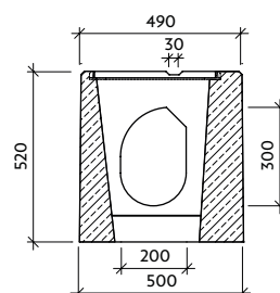
Řez: b-b'
