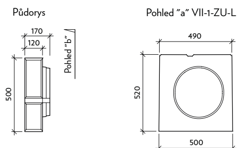
VII-1-ZU-L - záslepka pero levá
