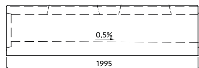
Profil VII-1-G27/28-L s vnitřním spádem
