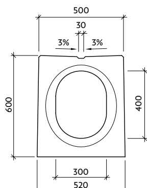
Pohled "a"="b" III-1-VU - drážka/drážka
