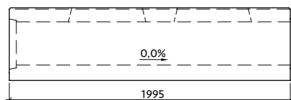
Profil VII-1-T30/30-L bez vnitřního spádu
