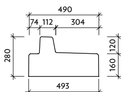
Pohled "a" VII-3-O
