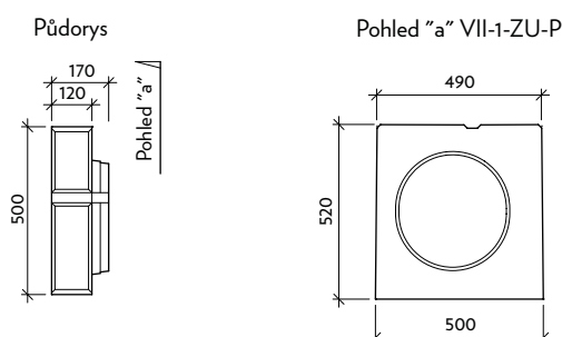
VII-1-ZU-P - záslepka pero pravá
