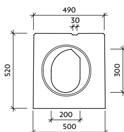
Pohled "b" VII-1-V0-P - pero
