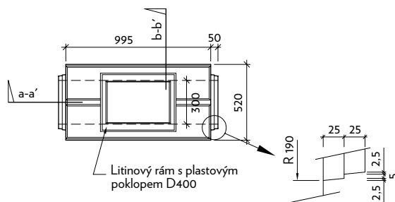
Půdorys
