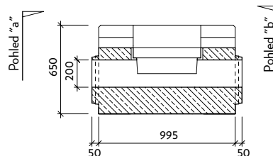
Řez: a-a' I-4-CS
