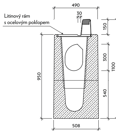
Řez: b-b' VII-4-PP-P
