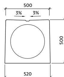
Pohled "b" II-ZU - drážka
