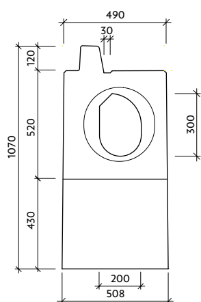
Pohled "a" VII-3-PP-P - drážka
