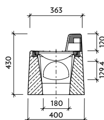
Řez: b-b' T-3-V0
