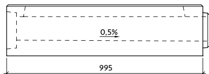
Profil M-G 120/125 se spádem dna
