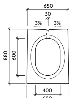
Pohled "a"="b" VI-1-VU - drážka/drážka
