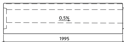
Profil VII-3-G22/23-P s vnitřním spádem
