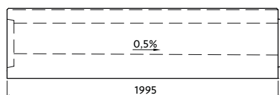
Profil VII-4-G28/29-L s vnitřním spádem
