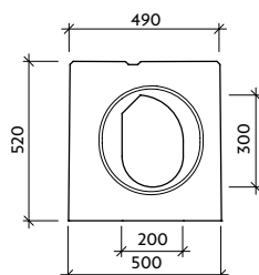
Pohled "b" VII-0-C0-L - pero
