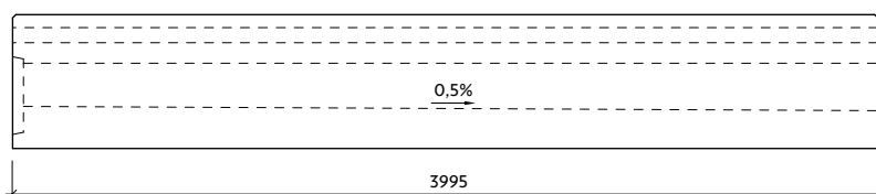
Profil I-5-G20/22-P se spádem dna
