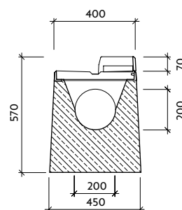
Řez: b-b' I-2-CS
