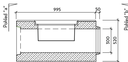
Řez: a-a' VII-I-C0-L
