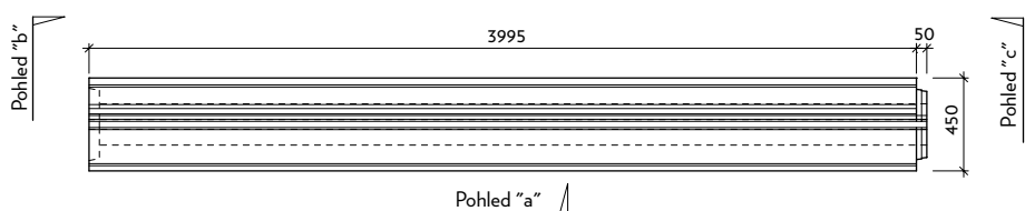
Půdorys
