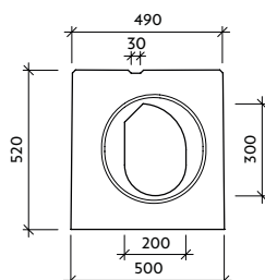
Pohled "b" VII-0-V0-L - pero
