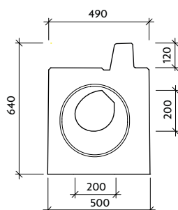
Pohled "b" VII-3-CS - pero
