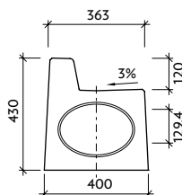
Pohled "a" T-3-ZU
