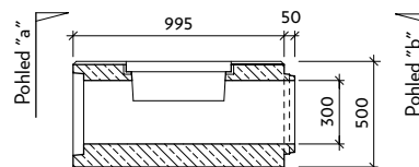
Řez: a-a' II-1-C0
