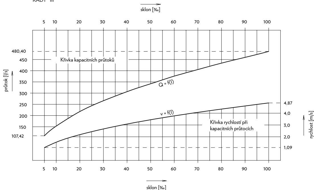
NOMOGRAM č. 1
