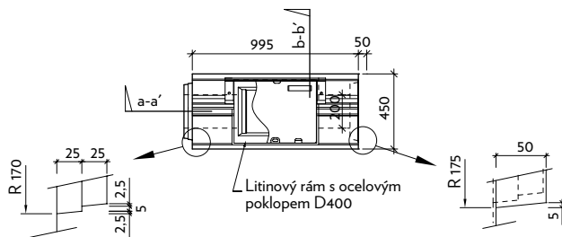
Pūdorys
