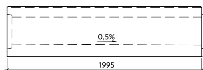
Profil VII-3-G28/29-L s vnitřním spádem
