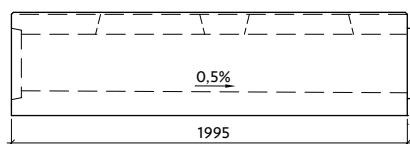
Profil VII-1-G29/30-P s vnitřním spádem
