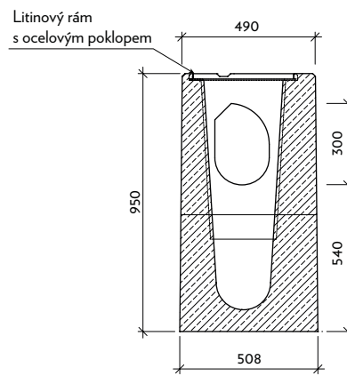
Řez: b-b' VII-1-PP-L
