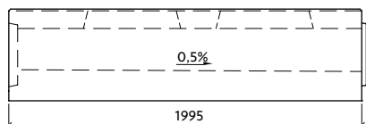
Profil VII-1-G23/24-P s vnitřním spádem
