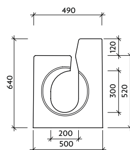
Pohled "c" - pero
