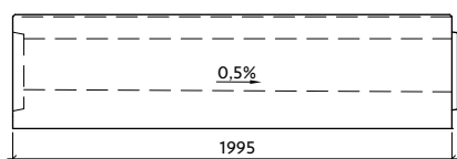
Profil VII-3-G23/24-P s vnitřním spádem
