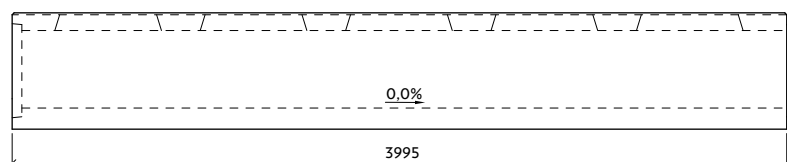
Profil III-1-T40/40 bez vnitřního spádu
