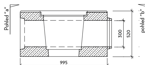
Řez: a-a' VII-1-V0-L
