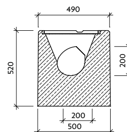
Řez: b-b'
