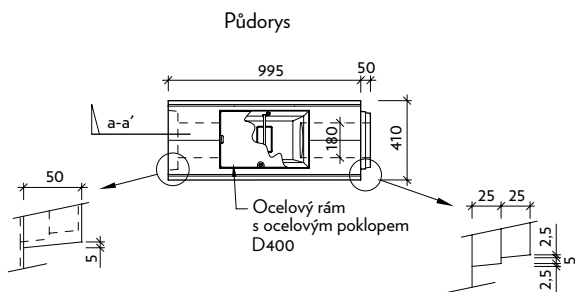
T-1-PP - bezpečnostní protipožární uzávěra s ocelovým poklopem pro zatížení D400
