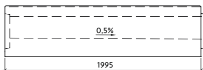
Profil VII-4-G22/23-P s vnitřním spádem
