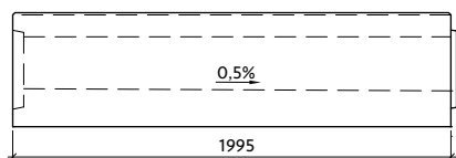
Profil VII-3-G24/25-P s vnitřním spádem
