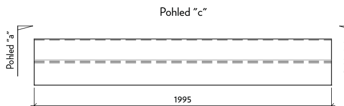
Profil VII-3-O tunelový obrubník
