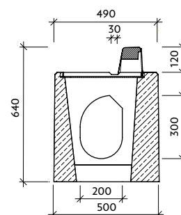
Řez: b-b'
