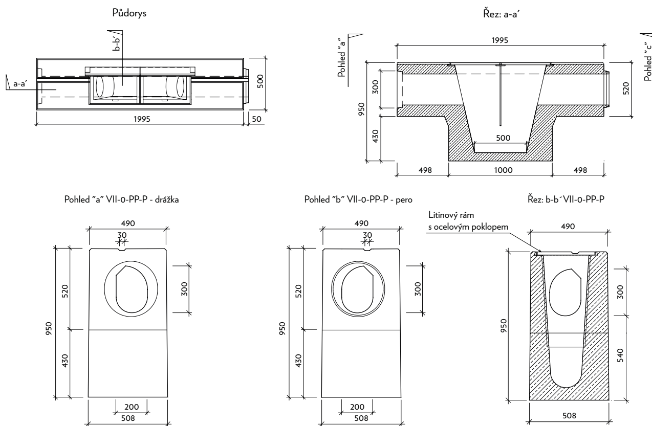
VII-0-PP bezpečnostní protipožární uzávěra
