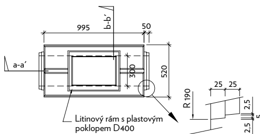
Půdorys
