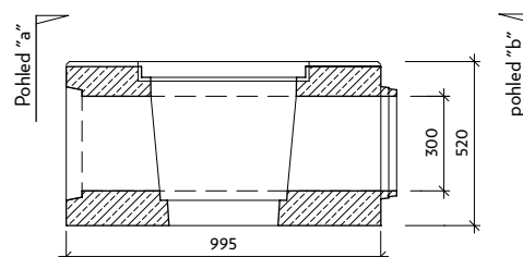
Řez: a-a' VII-1-V0-P
