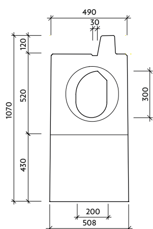
Pohled "a" VII-3-PP-L - drážka
