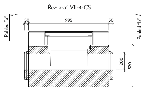
VII-4-CS čistící kus vrcholový
