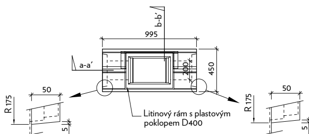
Půdorys
