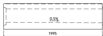
Profil VII-3-G27/28-L s vnitřním spádem
