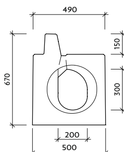
Pohled "a" VII-4-VU - drážka
