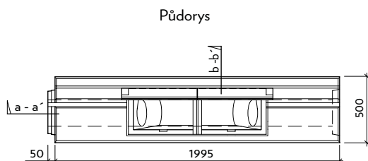
Profil VII-4-PP -pravý - bezpečnostní protipožární uzávěra
