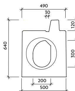
Pohled "b" VII-3-VU - drážka
