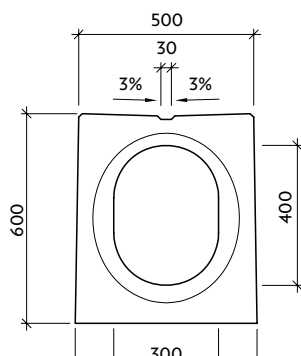
Pohled "a"="b" III-0-VU - drážka/drážka
