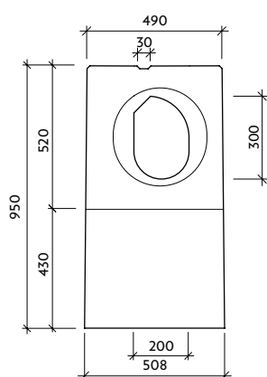
Pohled "a" VII-1-PP-P - drážka
