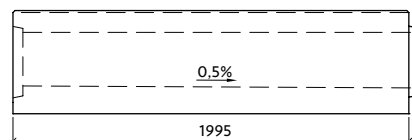
Profil VII-0-G27/28-L s vnitřním spádem
