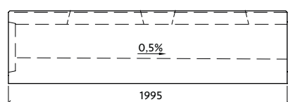
Profil VII-1-G23/24-L s vnitřním spádem
