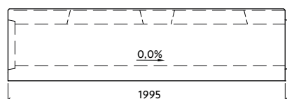
Profil VII-1-T30/30-P bez vnitřního spádu
