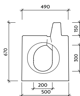
Pohled "b" VII-4-L-C0 - drážka
