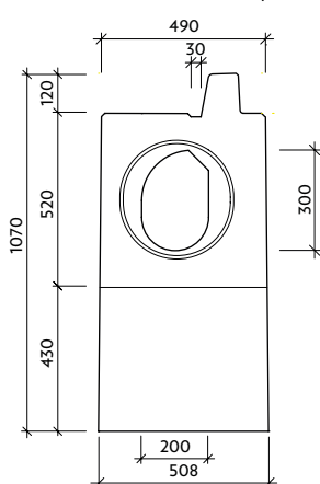
Profil VII-3-L - protipožární přepážka levá
