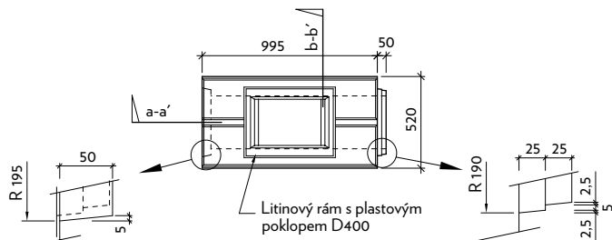
Pudorys
