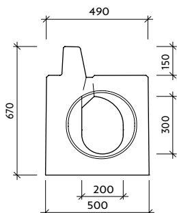
Pohled "a" V-4-L-V0 - pero
