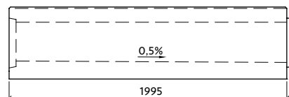
Profil VII-0-G28/29-L s vnitřním spádem
