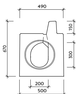
Pohled "b" VII-4-P-C0 - pero
