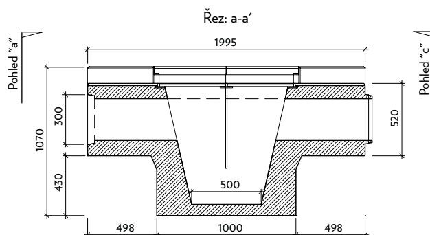
VII-3-PP bezpečnostní protipožární uzávěra
