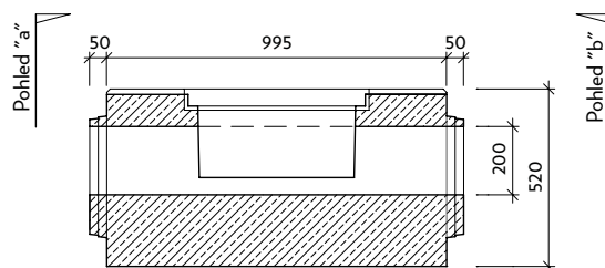
Řez: a-a' VII-I-CS
