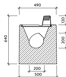
Řez: b-b'
