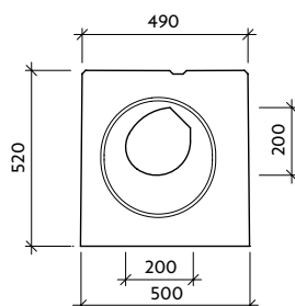
Pohled "b" VII-I-CS - pero
