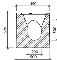
Řez: b-b'
