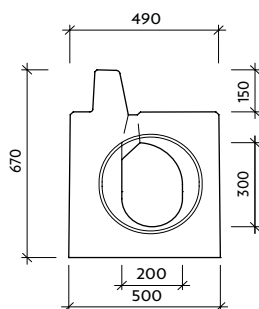
Pohled "a" VII-4-L-C0 - pero
