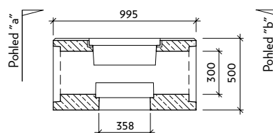
Řez: a-a'
