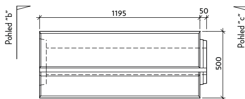
Podélný řez
