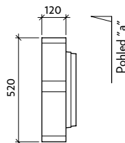
Pohled "a" III-ZU - pero
