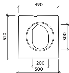
Pohled "b" VII-I-C0-L - pero
