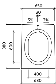
Pohled "a" VI-1-C0 - drážka
