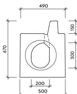
Pohled "b" VII-4-VU - drážka
