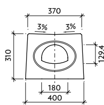
Pohled "b" T-0-V0 - pero
