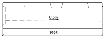
Profil VII-1-G26/27-P s vnitřním spádem
