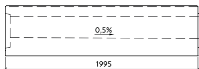
Profil VII-4-G22/23-P s vnitřním spádem
