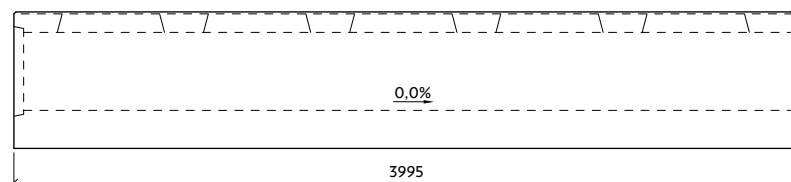
Profil IV-1-T40/40 bez vnitřního psádu
