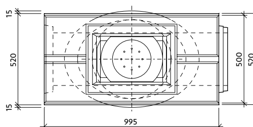
Půdorys
