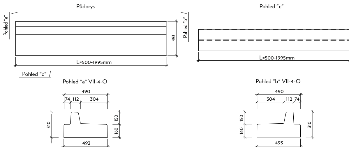
Profil VII-4-0 - tunelový obrubník
