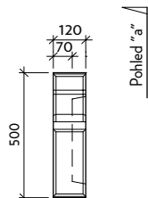
Půdorys VII-4-ZZ - levý
