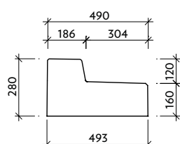
Pohled "b" VII-3-O-12-0
