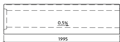
Profil VII-4-G29/30-L s vnitřním spádem
