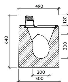
Řez: b-b'
