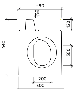
Pohled "a" VII-3-VU - drážka
