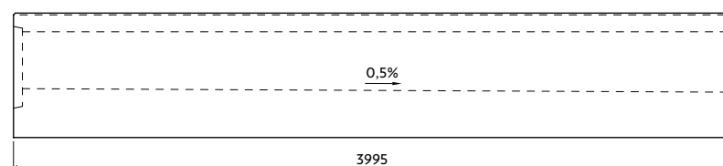
Profil IV-0-G32/34 se spádem dna
