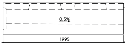
Profil VII-1-G24/25-P s vnitřním spádem
