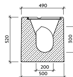
Řez: b-b'
