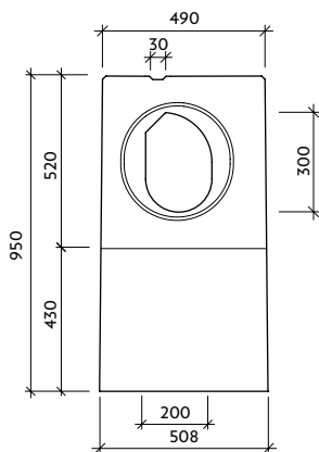
Pohled "b" VII-1-PP-L - pero
