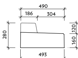
Pohled "a" VII-3-O-0-12
