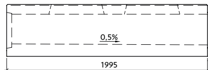
Profil VII-1-G29/30-L s vnitřním spádem
