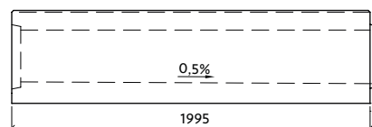
Profil VII-0-G24/25-L s vnitřním spádem
