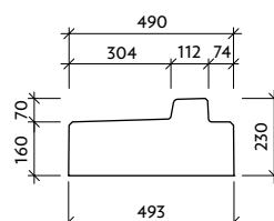
Pohled "b" VII-2-O
