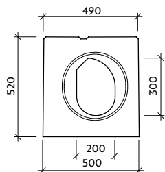
Pohled "b" VII-1-C0-L - pero
