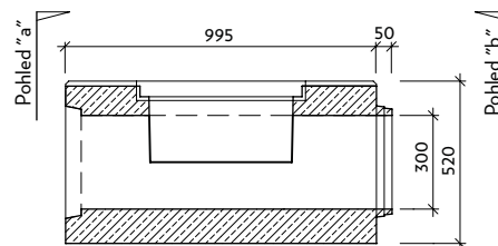
Řez: a-a' VII-1-C0-P
