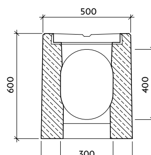
Řez: b-b'
