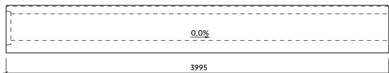
Profil I-0-T28/28 bez vnitřního spádu
