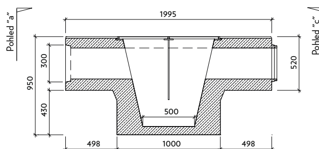
Pohled "b" VII-1-PP-P - pero
