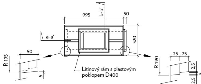
Půdorys
