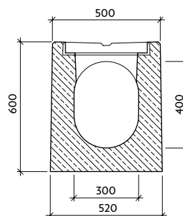
Řez: b-b'
