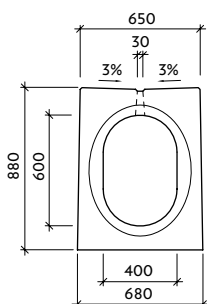
Pohled "a" VI-1-V0 - drážka
