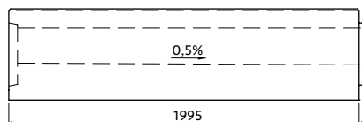
Profil VII-4-G20/21-L s vnitřním spádem
