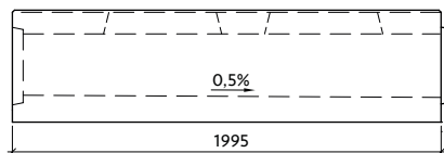
Profil VII-1-G29/30-P s vnitřním spádem
