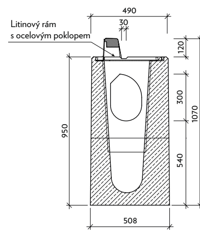
Řez: b-b' VII-3-PP-L
