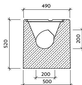
Řez: b-b'
