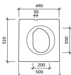
Pohled "a" VII-0-V0-P - drážka
