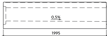
Profil VII-0-G20/21-L s vnitřním spádem
