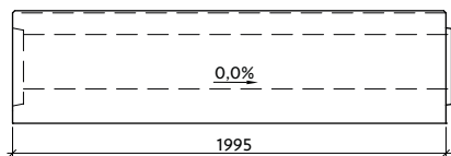
Profil VII-3-G25/26-P s vnitřním spádem
