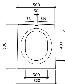
Pohled "a" III-0-C0 - drážka
