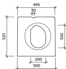
Pohled "a" VII-1-V0-P - drážka
