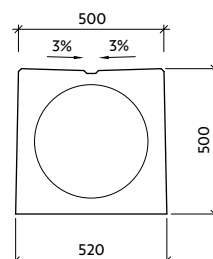
Pohled "b"
