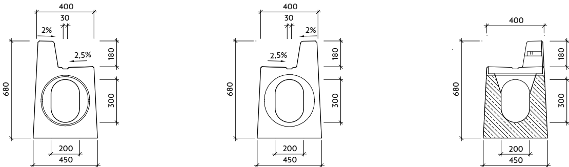
Pohled "a" I-7-C0 - pero
