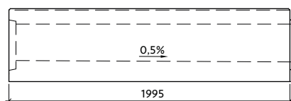
Profil VII-4-G26/27-L s vnitřním spádem
