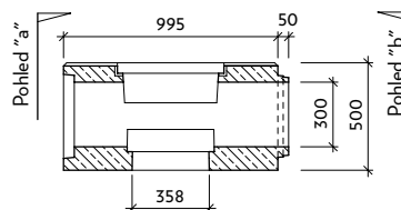
Řez: a-a' II-1-V0
