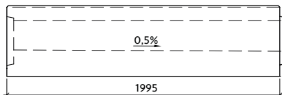
Profil VII-4-G21/22-L s vnitřním spádem
