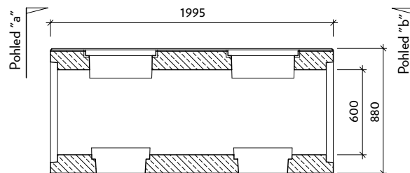
Řez: a-a'
