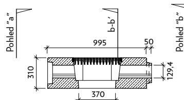
Řez: a-a' T-1-V0
