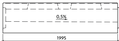
Profil VII-1-G22/23-P s vnitřním spádem
