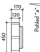
Půdorys T-ZU - levý
