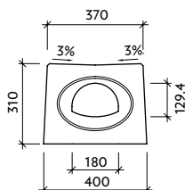
T-1-VU - vpustový kus úžlabí s litinovou mříží pro zatížení D400
