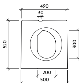
Pohled "a" VII-I-VU - drážka
