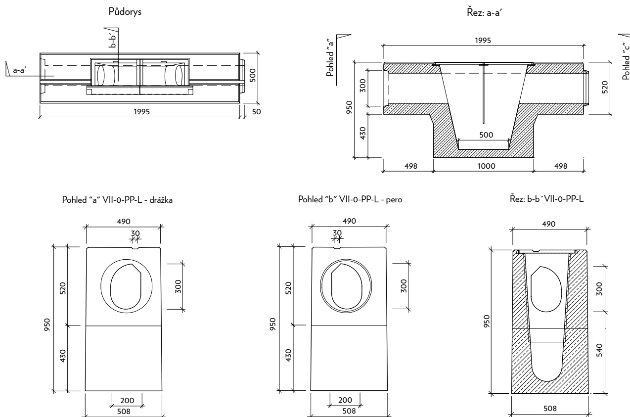
Profil VII-0-L - protipožární přepážka levá
