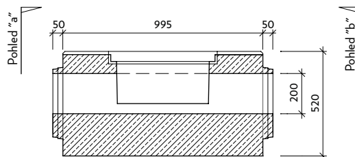
Řez: a-a' VII-0-CS
