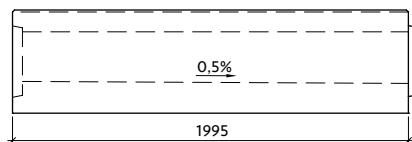
Profil VII-0-G24/25-P s vnitřním spádem
