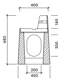
Řez: b-b' I-7-V0
