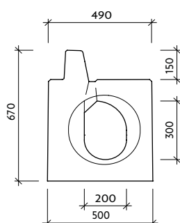
Pohled "a" VII-4-P-C0 - drážka
