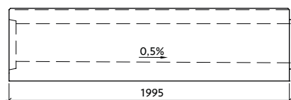
Profil VII-3-G27/28-P s vnitřním spádem
