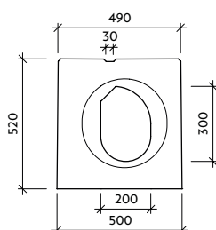
Pohled "a" VII-0-V0-P - drážka
