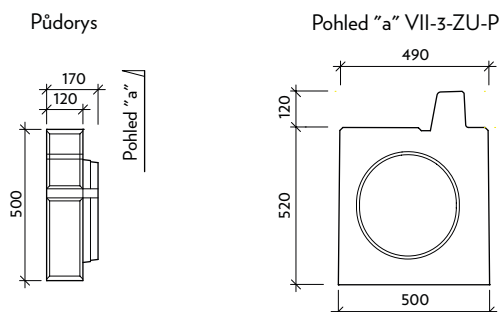
VII-3-ZU-P - záslepka pero pravá
