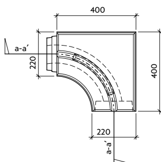
Půdorys
