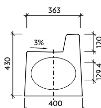
Pohled "a" T-3-ZZ
