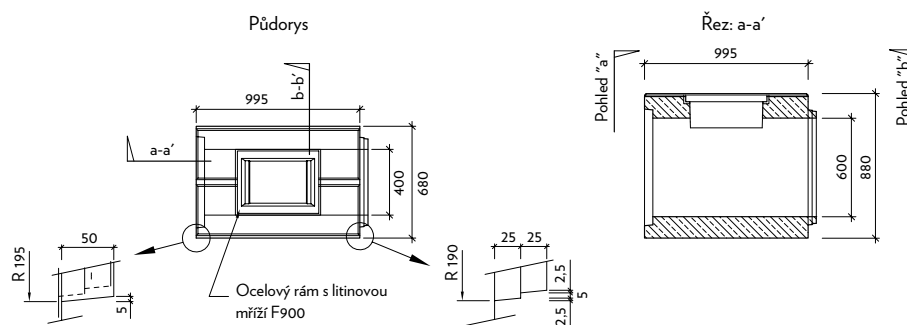
VI-1-C0 - čistící kus základní s ocelovým rámem a mříží pro zatížení F900
