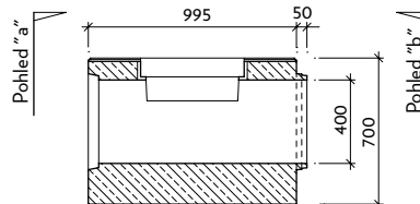
Řez: a-a' IV-1-C0
