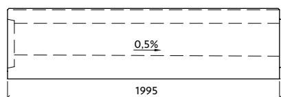
Profil VII-4-G23/24-P s vnitřním spádem
