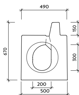
Pohled "b" VII-4-L-C0 - drážka
