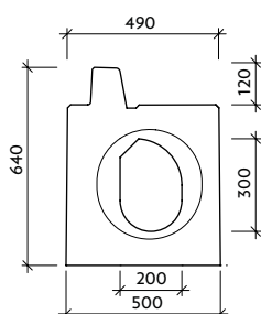
Pohled "a" VII-3-C0-P - drážka
