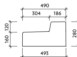
Pohled "b" VII-3-O-0-12
