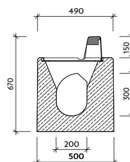
Řez: b-b'
