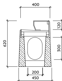
Řez: b-b' I-5-V0
