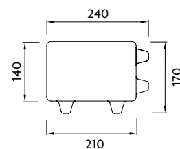
ukázka - půdorys
