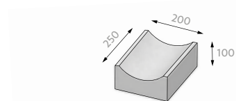
žlabovka 20
