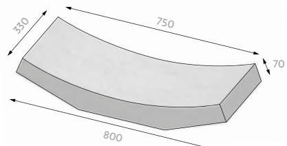
žlabovka 75
