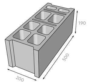
Zdicí tvárnice k půlení
