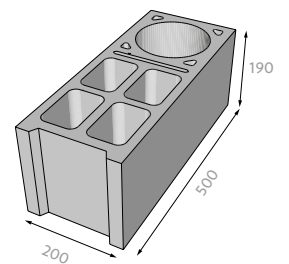
Zdicí tvárnice rohová
