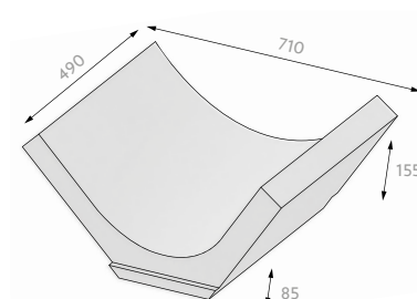
žlabovka svahová
