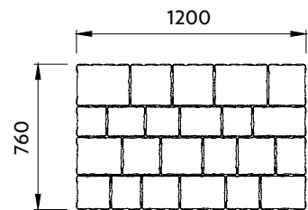
skladba na paletě
