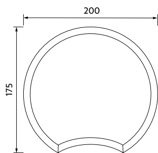
ukázka - půdorys
