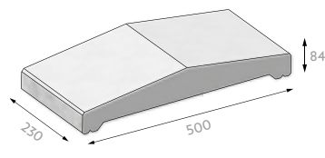
stříška 40 štípaná
