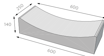
žlabovka - rovné hrany NOVINKA!
