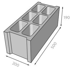
Zdicí tvárnice základní
