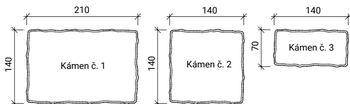
Půdorys
