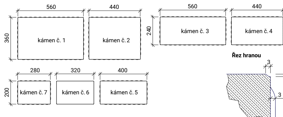
Půdorys
