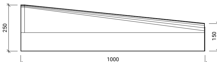
Obrubník nájezdový H 15
