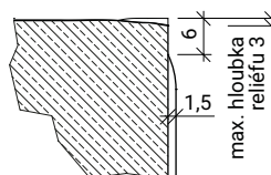
Řez hranou
