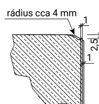
Řez hranou (v 60 mm)
