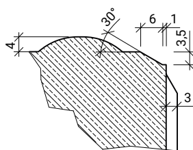
Řez hranou (v 80 mm)
