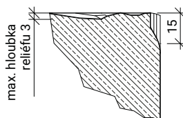
Řez hranou
