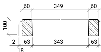
Řez: a - a'
