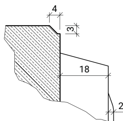
Řez hranou
