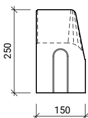
Pohled zprava
