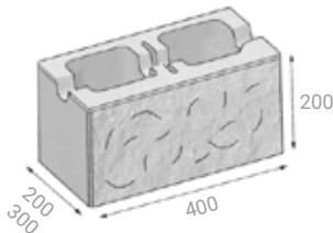
jedostranně štípaný k půlení s prolisem na výztuž
