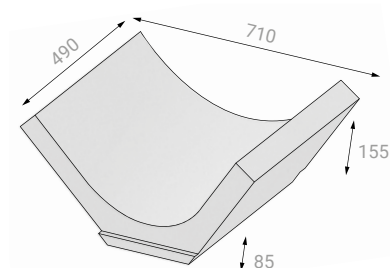
žlabovka svahová ukázka tvarů
