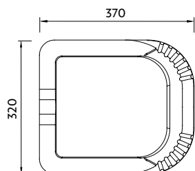
ukázka - půdorys
