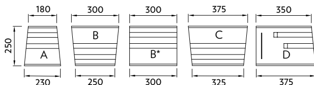
stříška – skladba 4 kamenů
