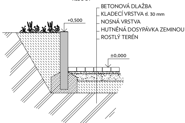
Řez a-a':
