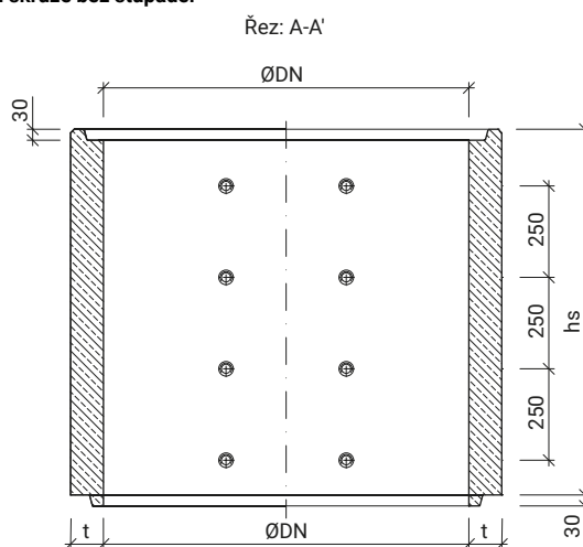
TBS-Q.2 Studniční skruže s žebříkovými stupadly
