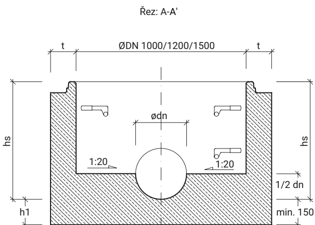
TBZ-Q.1 šachtové dno kompaktní jednolitě CAPITAN (kyneta 1/2)
