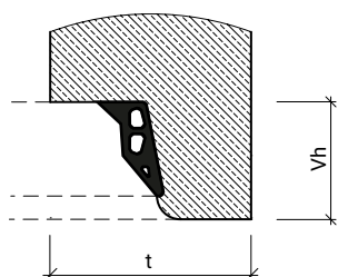
hrdlo - těsnění INTEGRO
