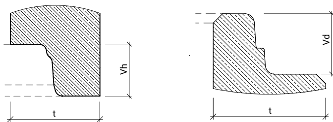
Detail tvaru hrdla a dříku TBS-Q.1
