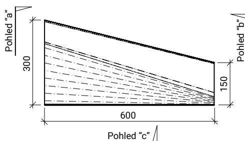
Půdorys
