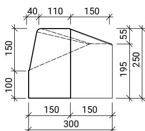
Pohled "b"
