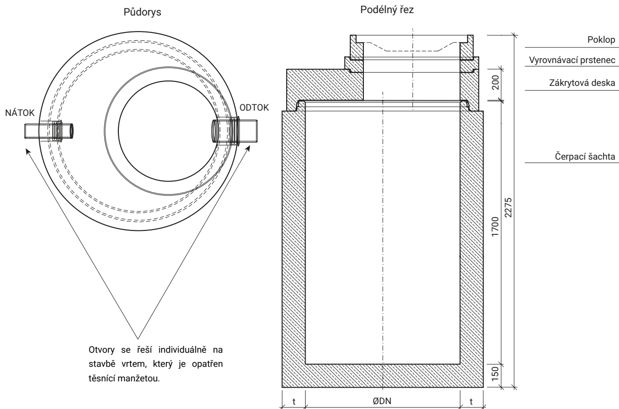
Čerpací šachta pro tlakovou kanalizaci
