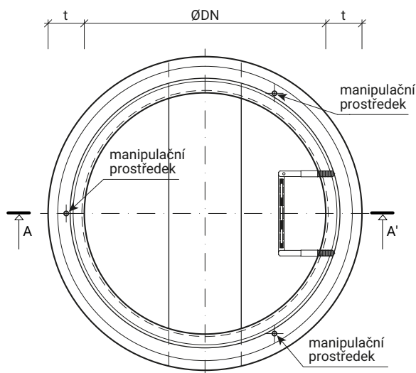
TBZ-Q.1 šachtové dno kompaktní jednolitě CAPITAN (kyneta 1/2)
