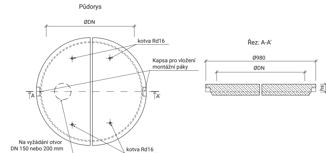
TZK-Q.2 Zákrytová deska DN 800 půlná
