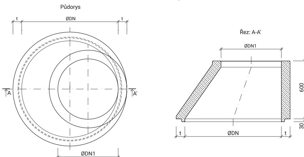
Detail dířku TBR-Q.2
