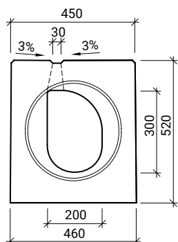
Čelní pohled
