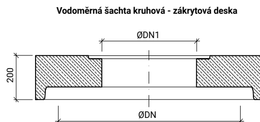
Podélný řez
