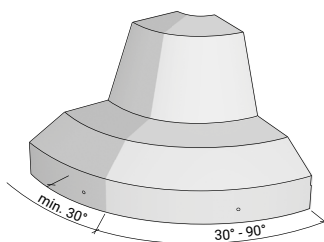
Obrubník odrazný rádius vnější R1 30°- 90°
