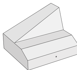
Obrubník odrazný polygonální rádius R4 - R25 vnitřní
