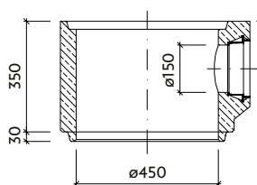
TBV-Q 450/350/3a PVC
