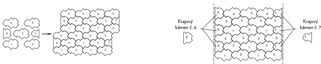
Pokládka dlažby CSB-CANTERA - využití krajových kamenů
