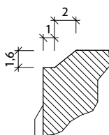
Řez hranou
