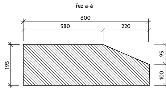
řez A-A
