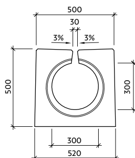
Pohled "a"="b" II-O-CS - pero/pero
