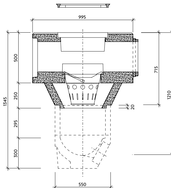
Řez a-a'
