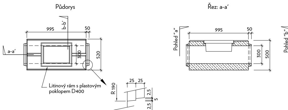
II-O-CS - čistící kus vrcholový s litinovým rámem a plastovým poklopem pro zatížení D400
