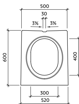
Pohled "b" III-O-C0 - pero
