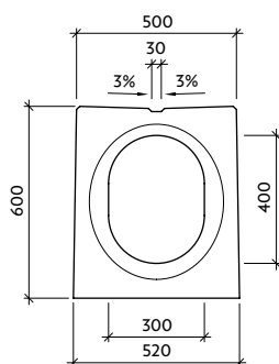
Pohled "a" III-1-V0 - drážka
