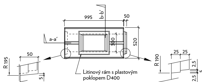
Pohled "a" III-1-V0 - drážka
