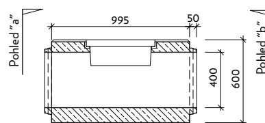
Řez: a-a'
