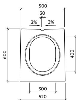
Pohled "b" III-O-V0 - pero
