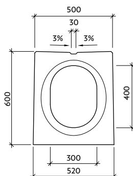
Pohled "a"="b" III-O-VU - drážka/drážka
