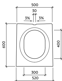
Pohled "a" III-O-C0 - drážka
