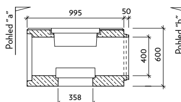
Řez: a-a' III-1-V0
