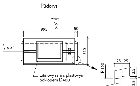
III-O-CS - čistící kus základní s litinovým rámem a plastovým poklopem pro zatížení D400
