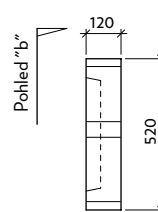
Pohled "b" III-ZZ - drážka
