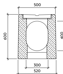
Řez: b-b' III-1-V0
