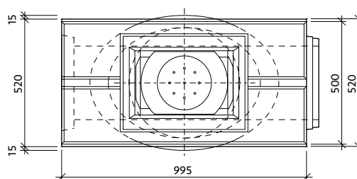
Půdorys
