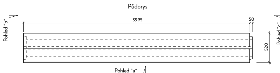
Profil III-O - štěrbinová trouba
