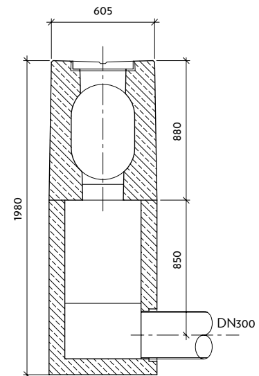
Řez: b-b'
