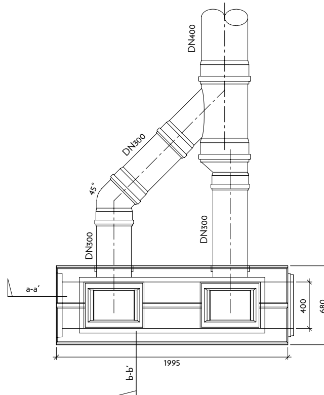
Půdorys
