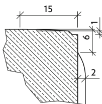
Řez hranou
